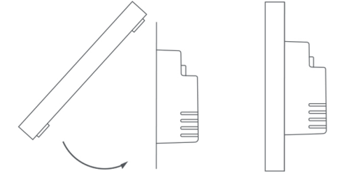
首先,面板斜向下,顶部向上卡槽,其次,面板下部直接下压扣合
